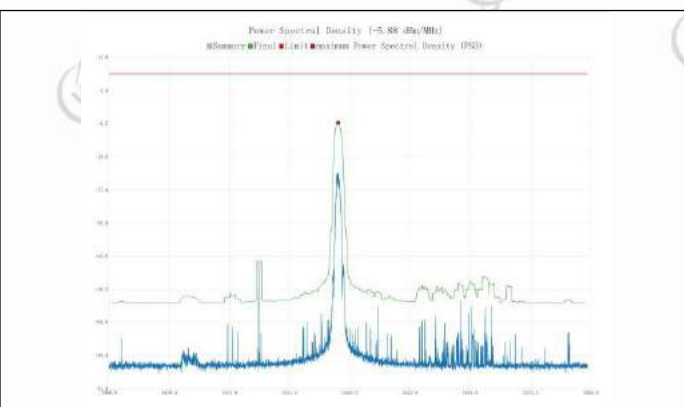
BLE 1M_Channel 19
