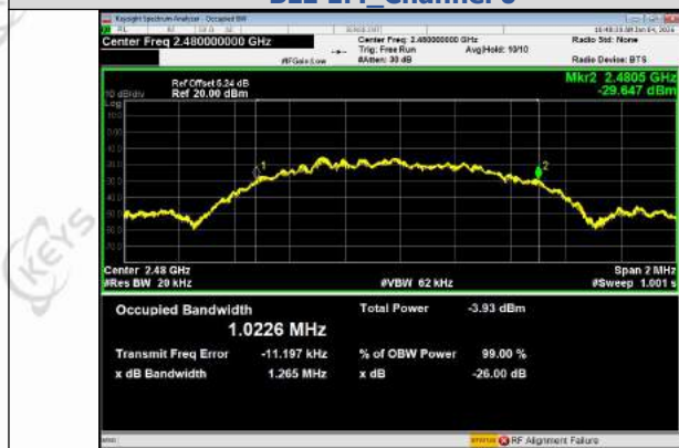
BLE 1M_Channel 39
